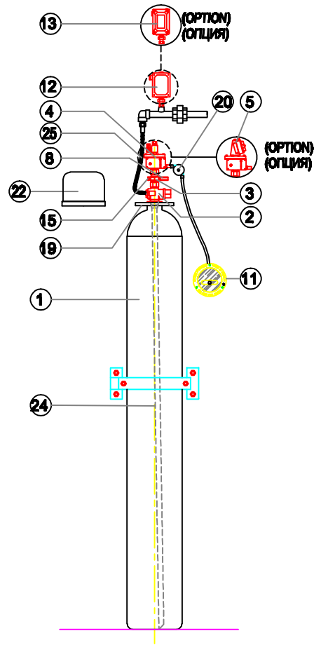
WEIGHTING SYSTEM ASSEMBLY (OPTIONAL) СИСТЕМА ВЗВЕШИВАНИЯ (ОПЦИЯ)
