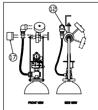
WEIGHTING SYSTEM ASSEMBLY (OPTIONAL) СИСТЕМА ВЗВЕШИВАНИЯ (ОПЦИЯ)
